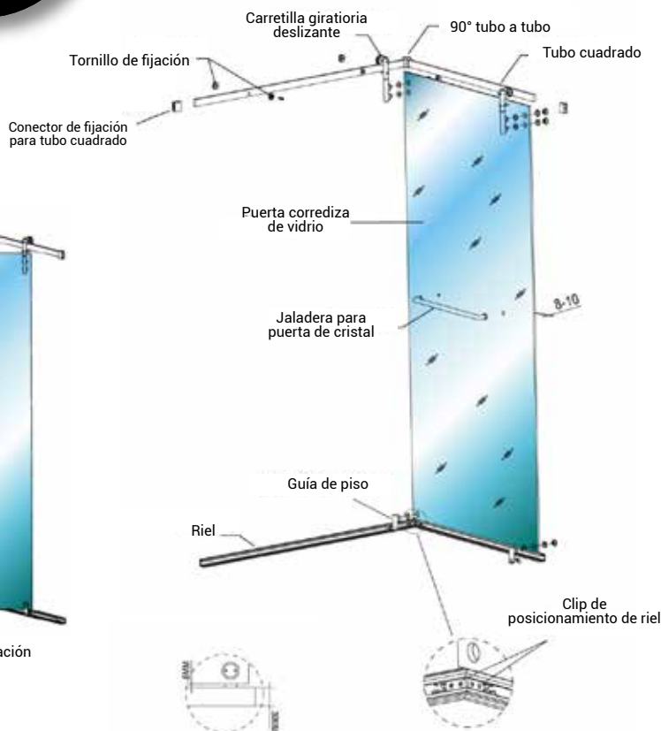
Instalación para mantener recta la guía de piso
